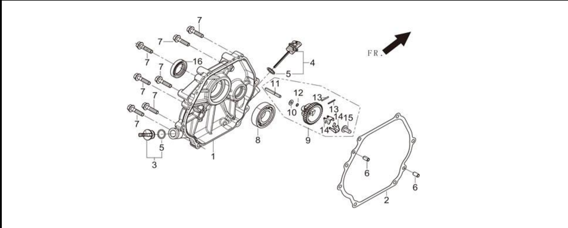
图3： 曲轴箱盖组合、调速齿轮部件（E01）
