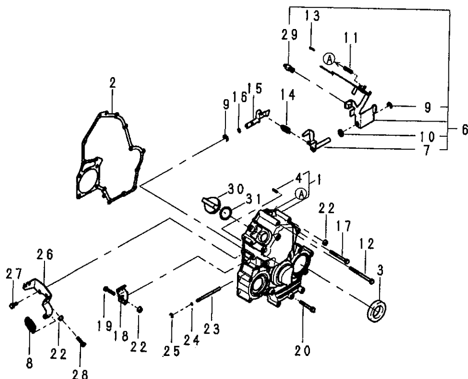
タイミングギヤ&ガバナー FIG.106 TIMING GEAR & GOVERNOR
