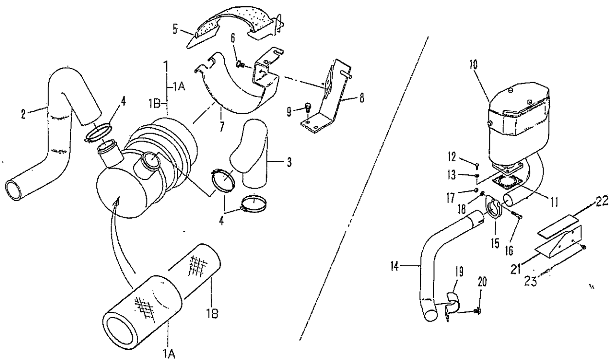
FIG.112 エアクリーナ, マフラ AIR CLEANER, MUFFLER
