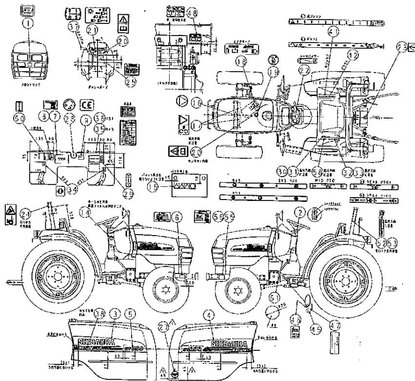
FIG.241 コーシヨンプレート CAUTION PLATE
