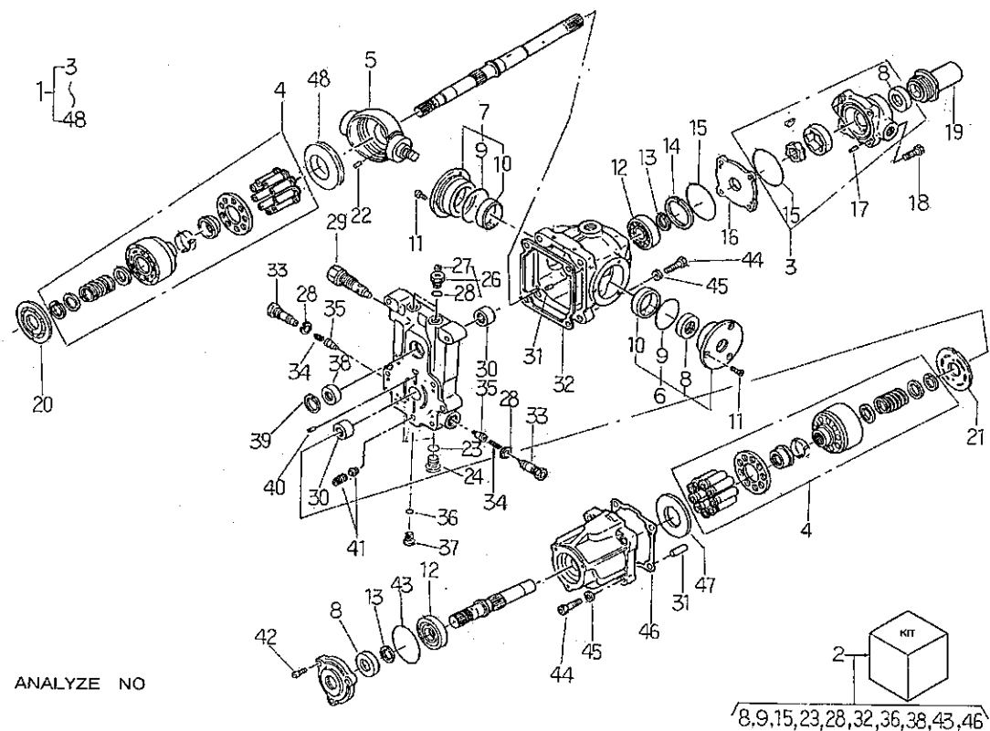
FIG.236 H. S. T. H. S. T
