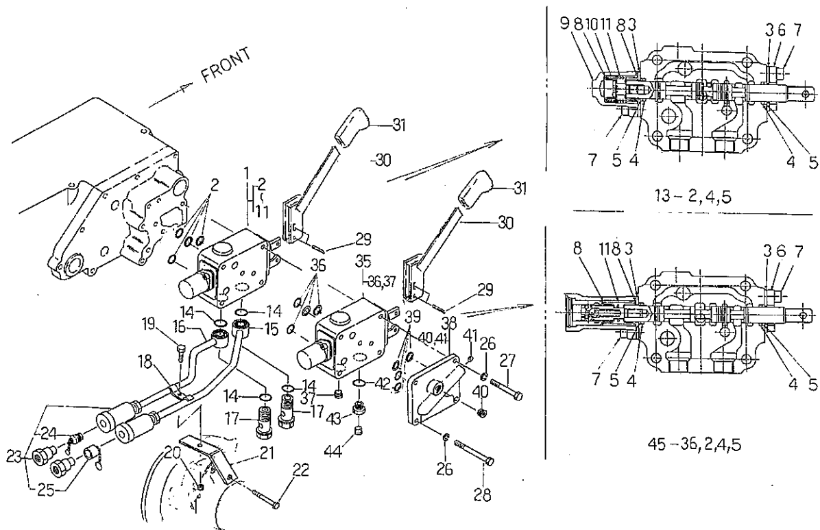
FIG.229 アタッチメントバルブ；二連 ATTACHMENT VALVE ; 2-SPOOL
