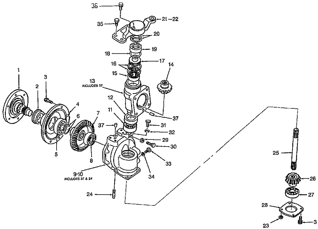
フロントアクスル; ファイナル FRONT AXLE ; FINAL
