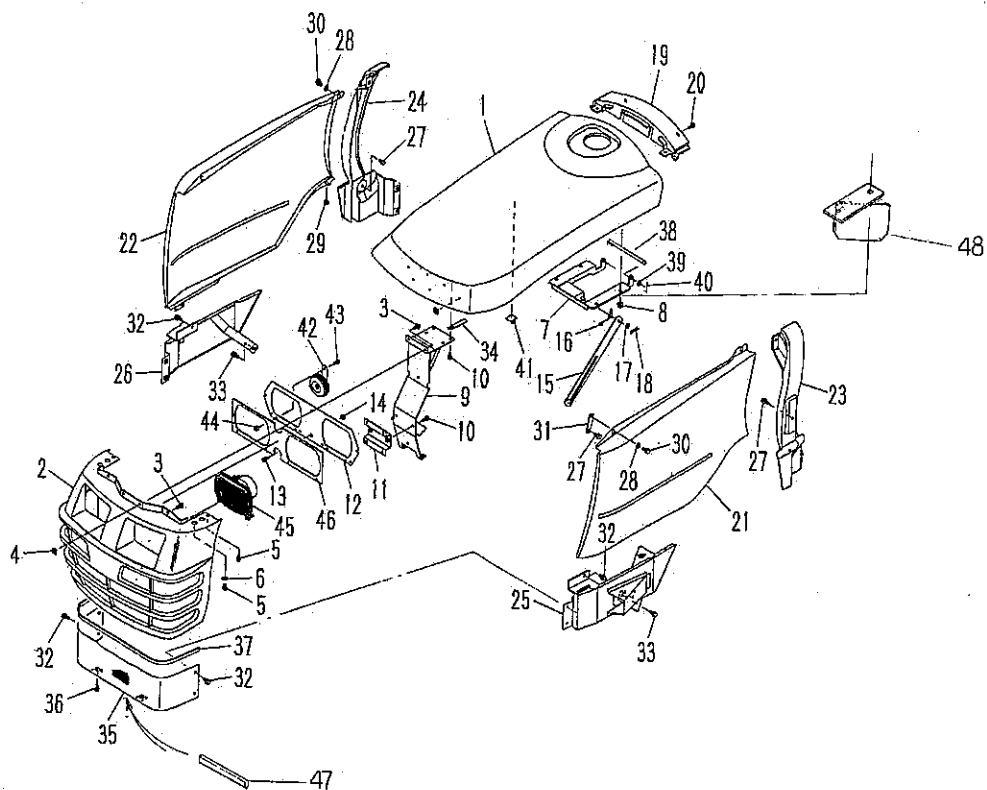
FIG.237 ボンネット BONNET
