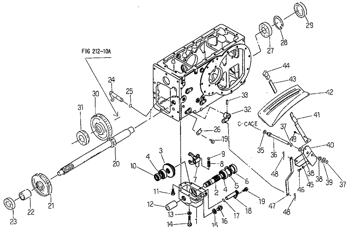
ミッド PTO FIG.211 MID P. T. O
