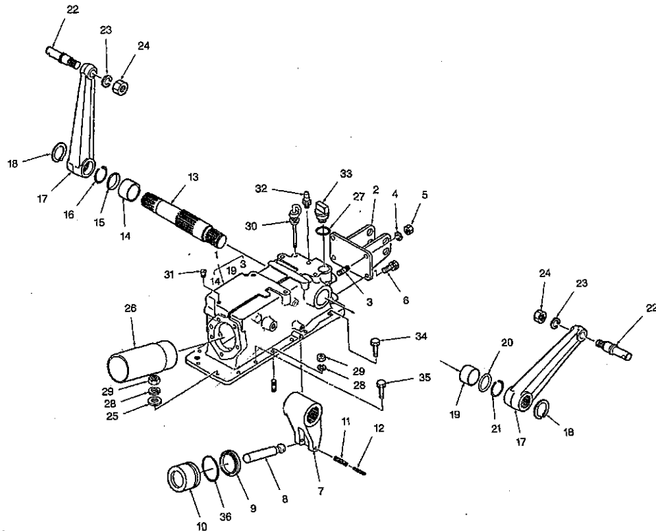
FIG.223 油圧シリンダ HYD-CYLINDER
