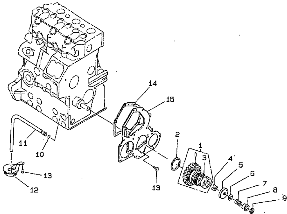
FIG.107 オイルポンプ OIL PUMP
