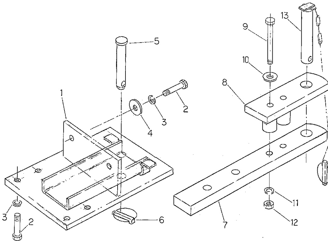
FIG.243 トレーラヒッチ TRAILER HITCH
