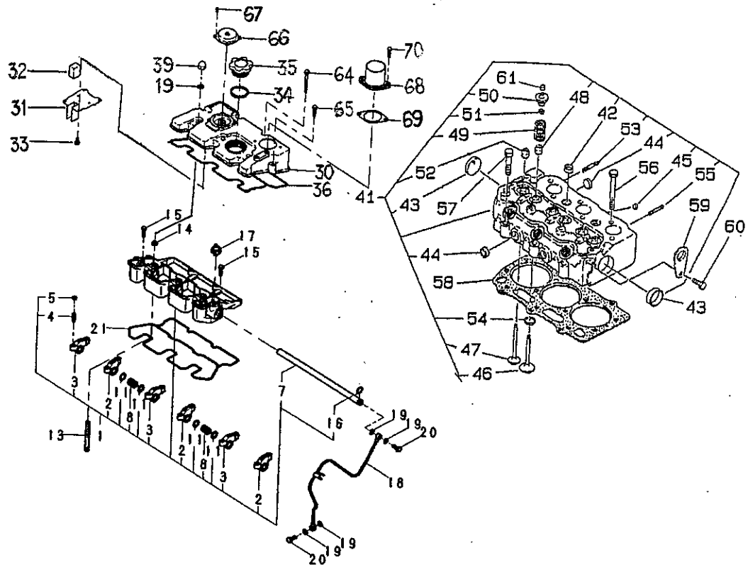
FIG.103 シリンダヘッド, ロッカアーム CYLINDER HEAD, ROKER ARM
