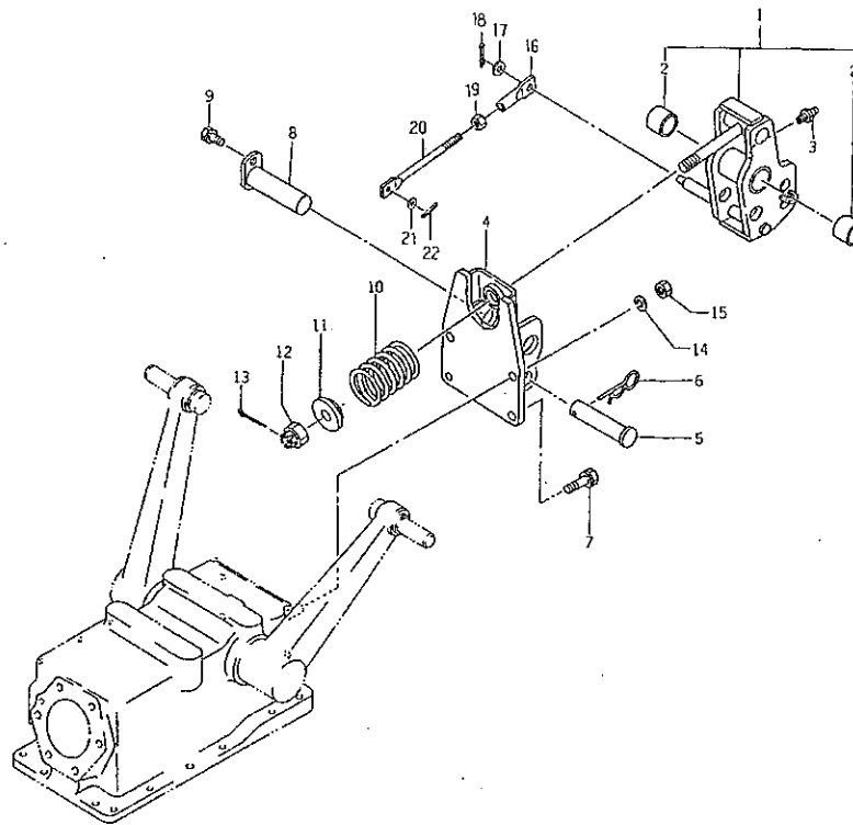
FIG.225 トップリンクブラケット TOP LINKE BRACKET
