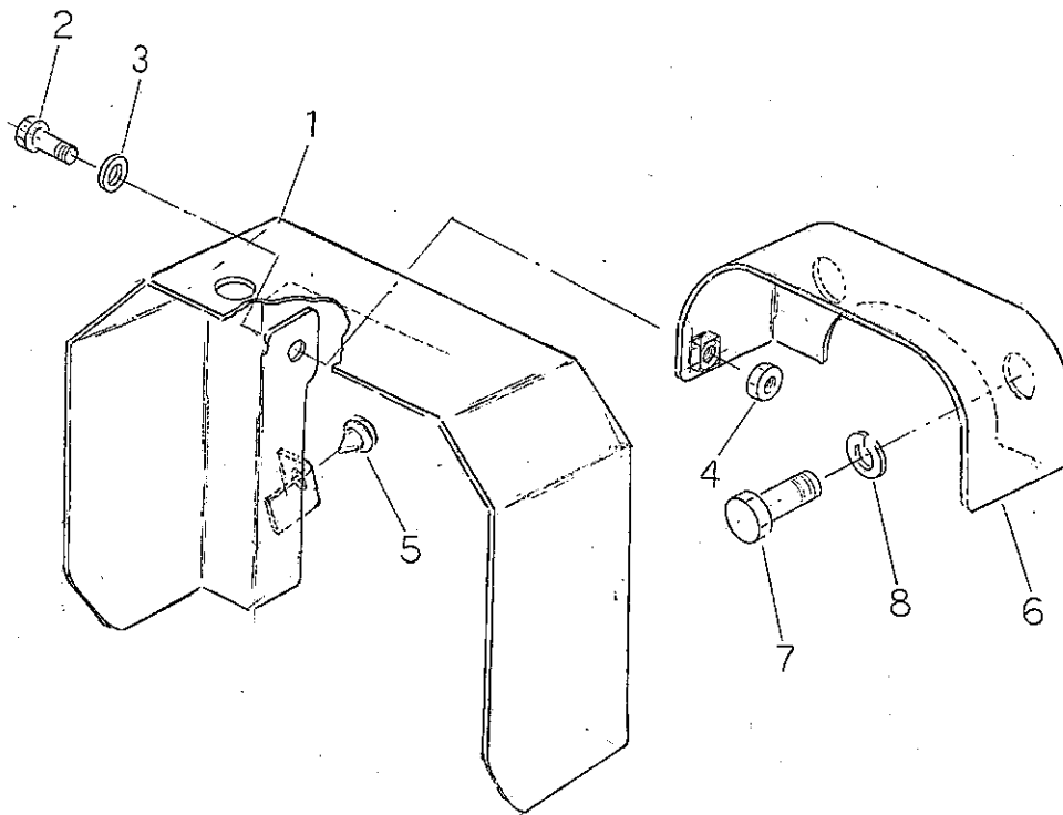
GUARD ; P. T. O
