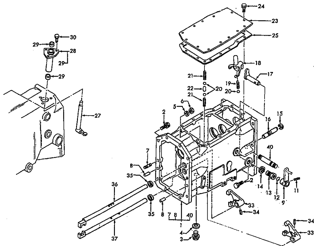
FIG.209 ミッション; 9×3 シフト MIDDLE MISSION ; SHIFT
