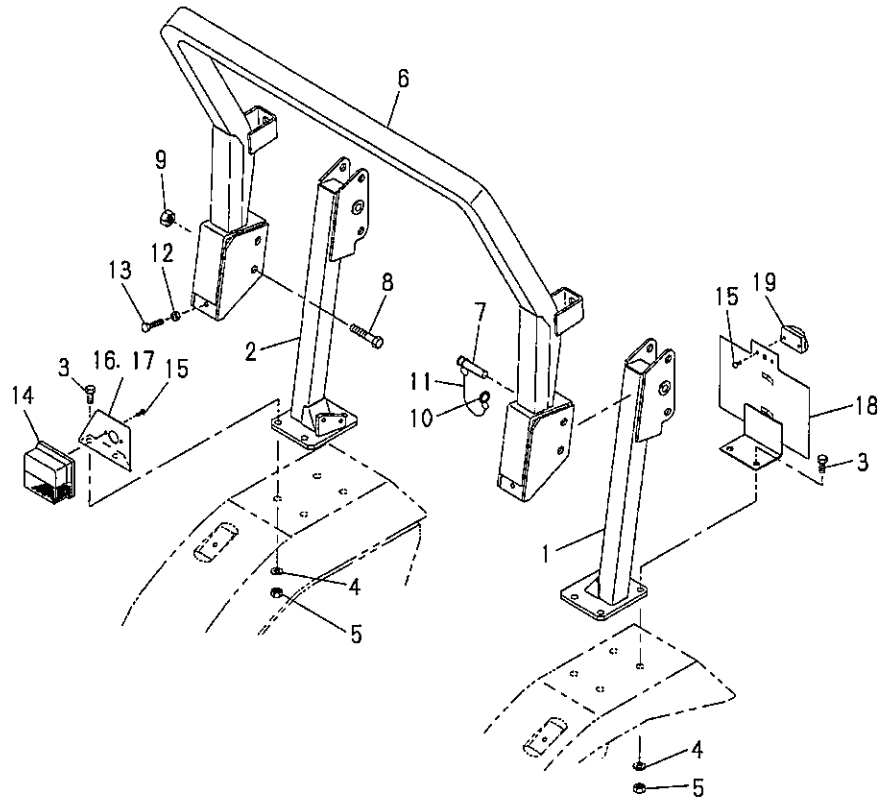
安全フレーム；上部 FIG.216 SAFETY FRAME ; UPPER
