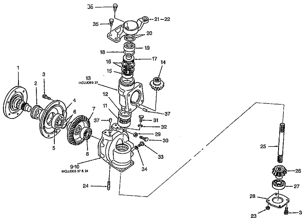
FIG.203 フロントアクスル；ファイナル FRONT AXLE ; FINAL
