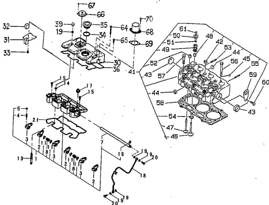
FIG.103 シリンダヘッド, ロッカーアーム CYLINDER HEAD, ROKER ARM
