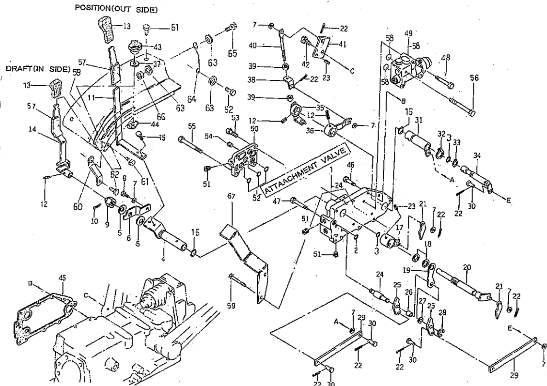
FIG.227 バルブカバー；ドラフト，ポジション付 VALVE COVER ; W/DRAFT, POSITION
