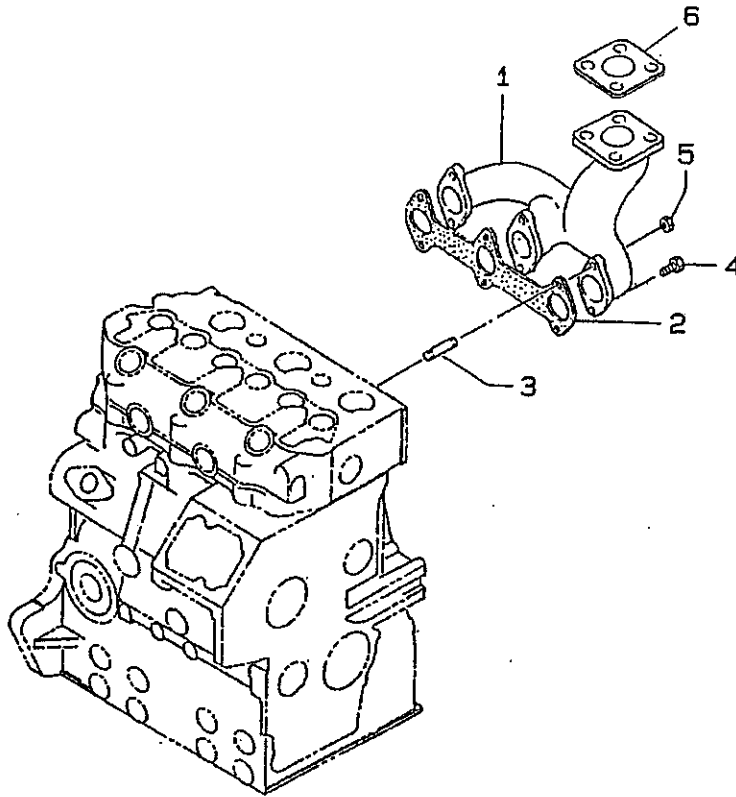
エグゾースト マニフォールド EXHAUST MANIFOLD ; EX
