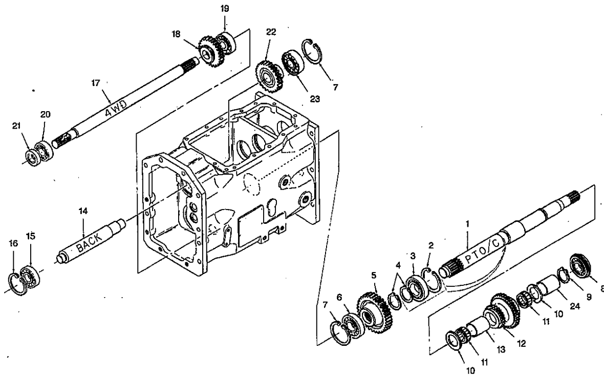
FIG.206 ミッション ; 9x3 4W PTO MIDDLE MISSION ; MECHA
