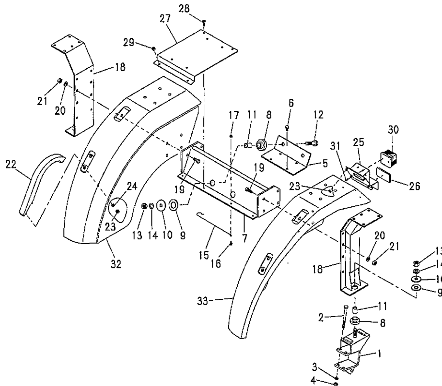
安全フレーム FIG.215 SAFETY FRAME
