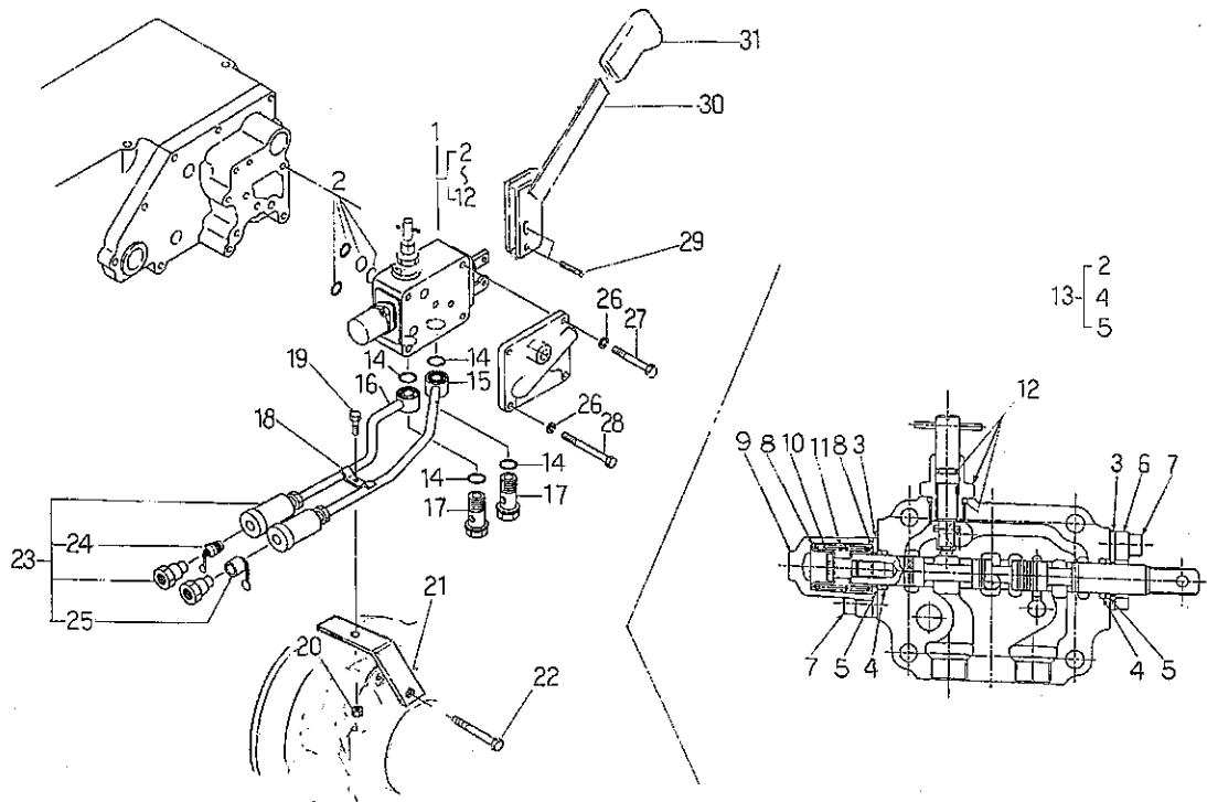
FIG.228 アタッチメントバルブ；一連 ATTACHMENT VALVE ; 1-SPOOL
