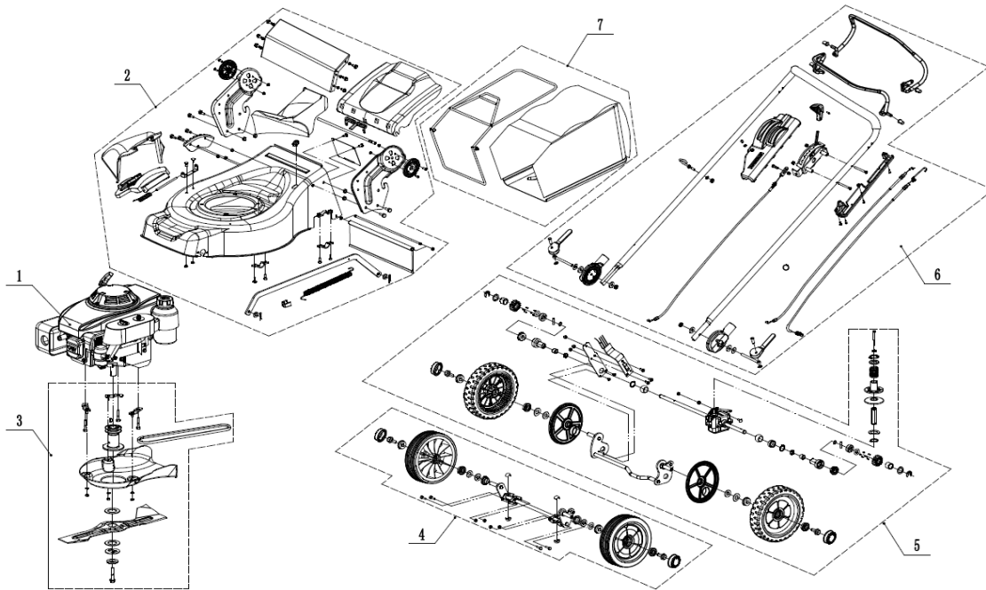
FIG.1 FERRO47HV Spare parts list
