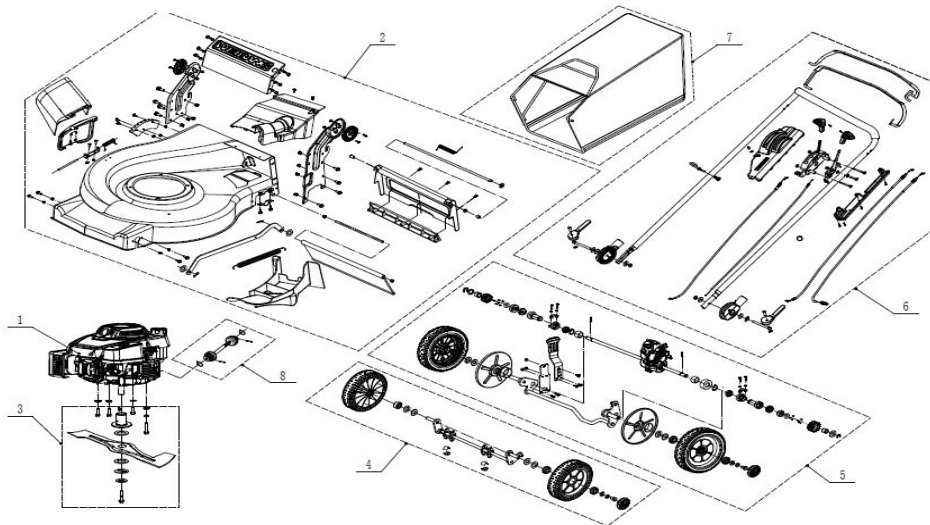
FIG.1 Ixo 52CV Spare parts list
